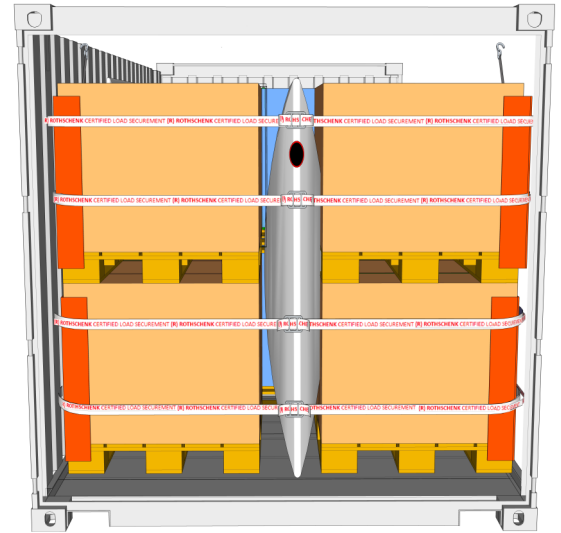
CP1 Palette 1.200 x 1.000 mm
